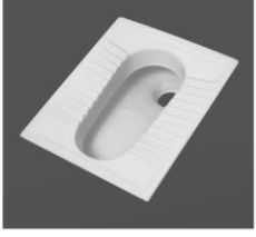
ORISSA PAN - 20" 510 x 410 x 260mm
