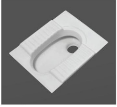
CT PAN - 20" 515 x 430 x 160mm
